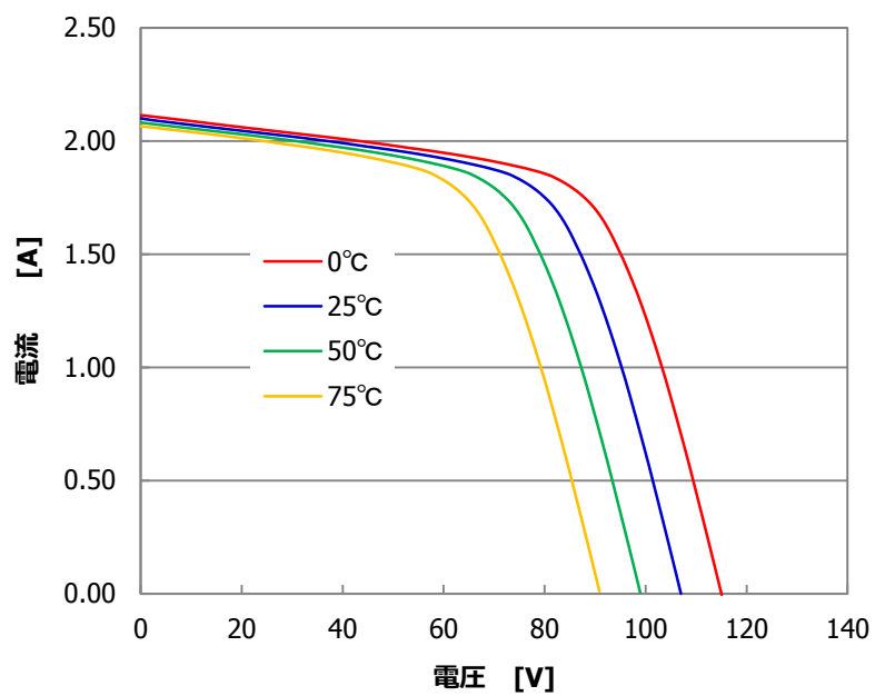
モジュール温度別 I-V 代表特性 型式：SF140-S 測定条件：AM1.5 1,000W/m 2
